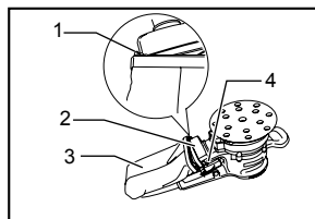
1. Crochet 2. Raccord à poussières 3. Sac à poussières 4. Bouton-poussoir
