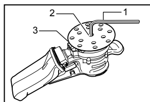
1. Clé hexagonale 2. Vis 3. Plateau
