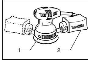
1. Skirt 2. Dust bag
