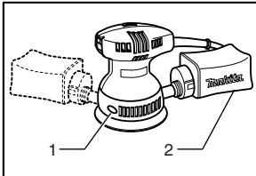
1. Jupe 2. Sac à poussières
