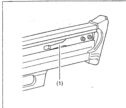
(1) Butée des clous
