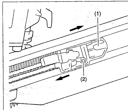
(1) Levier du poussoir (2) Poussoir
