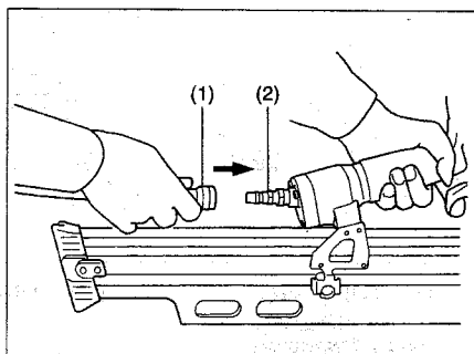
(2) Raccord d'air
